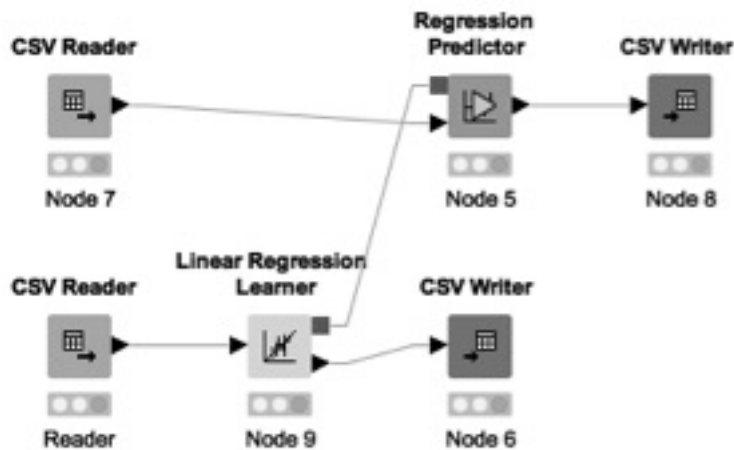
Рис. 1. Схема проекта Knime
